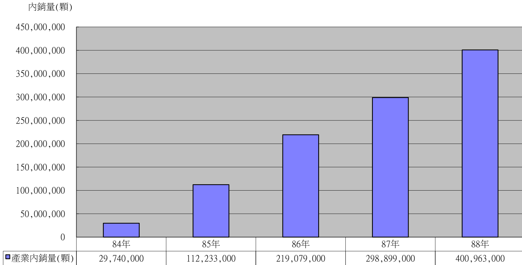
圖九 DRAM產業以顆計之內銷量趨勢圖
