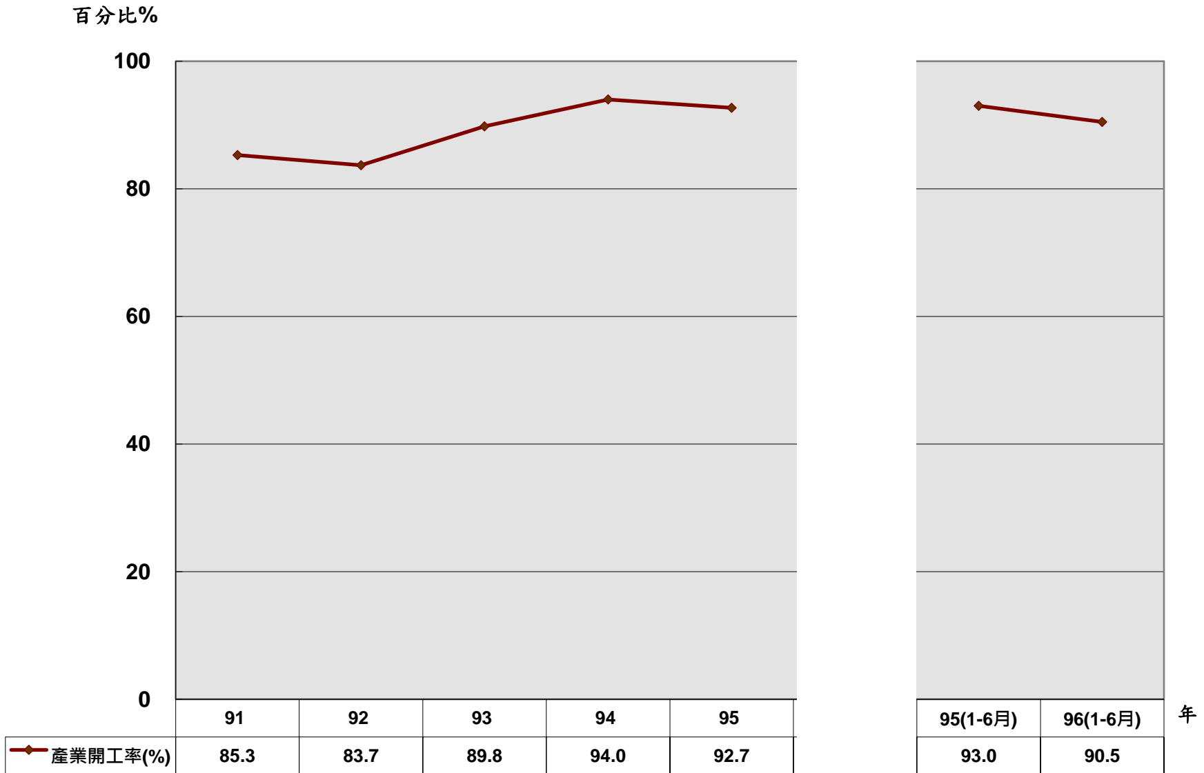
圖8 我國卜特蘭水泥暨其熟料產業產能利用率趨勢圖
