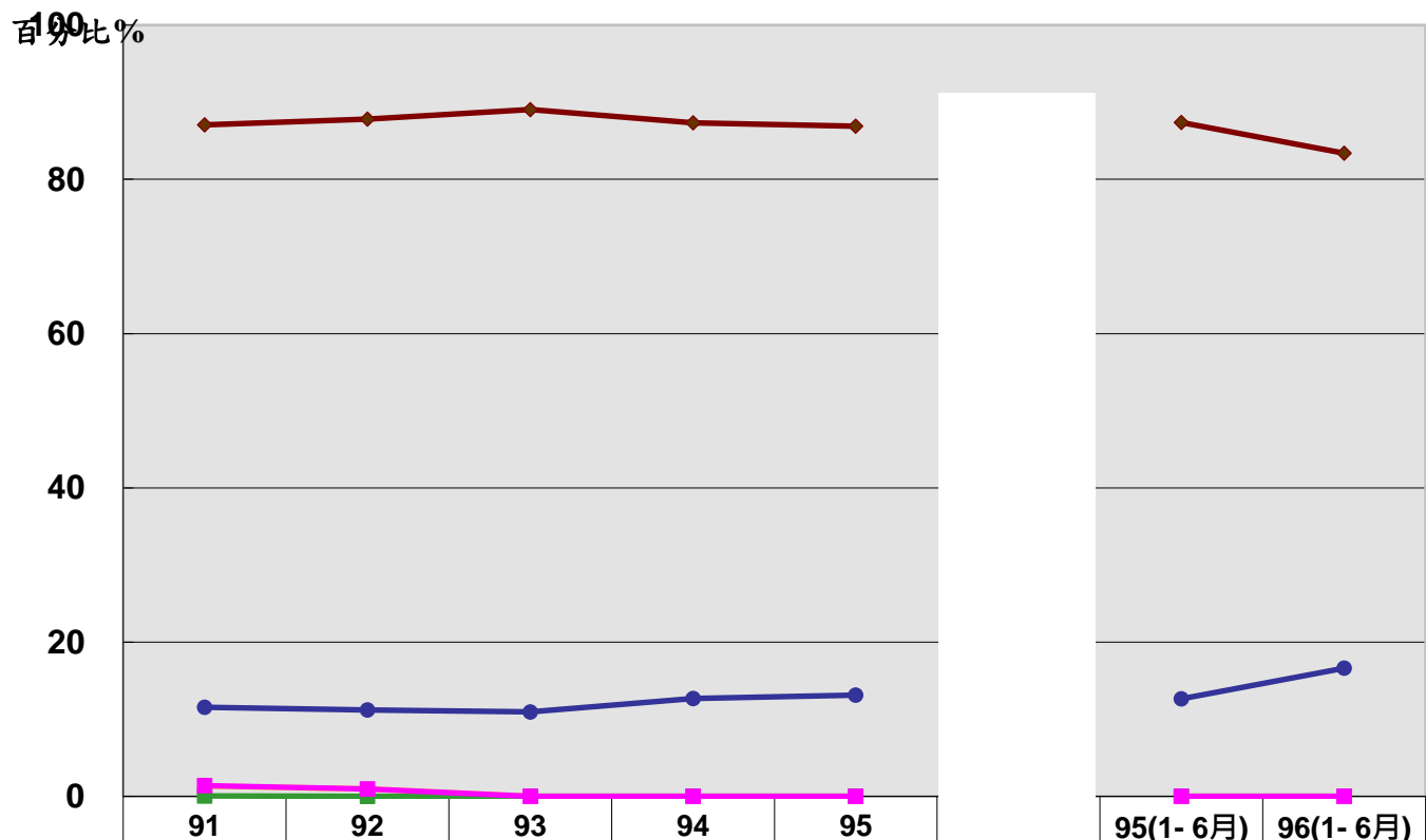
圖4 卜特蘭水泥暨其熟料進口量相對我國消費量趨勢圖
