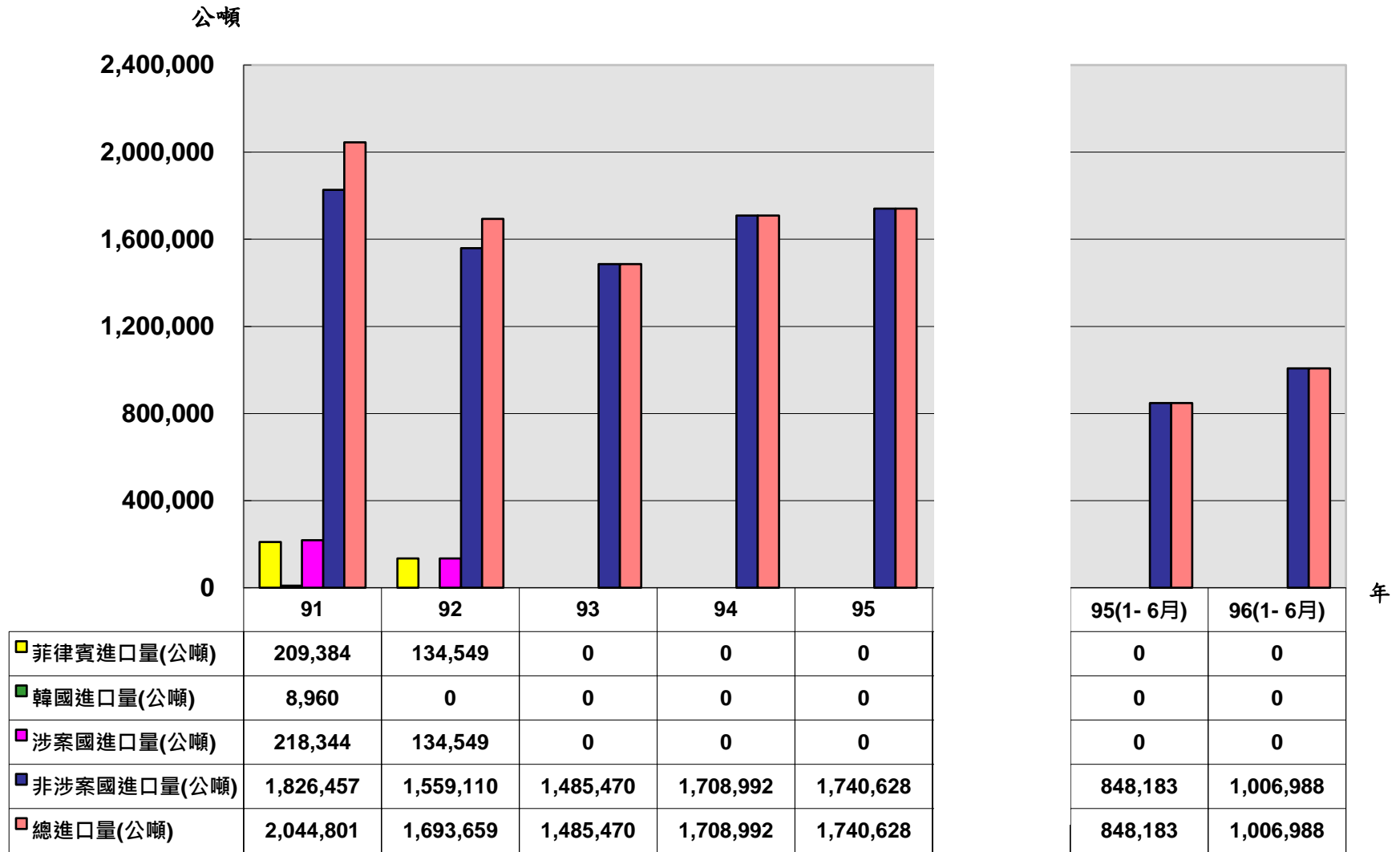
圖1 卜特蘭水泥暨其熟料進口量趨勢圖
