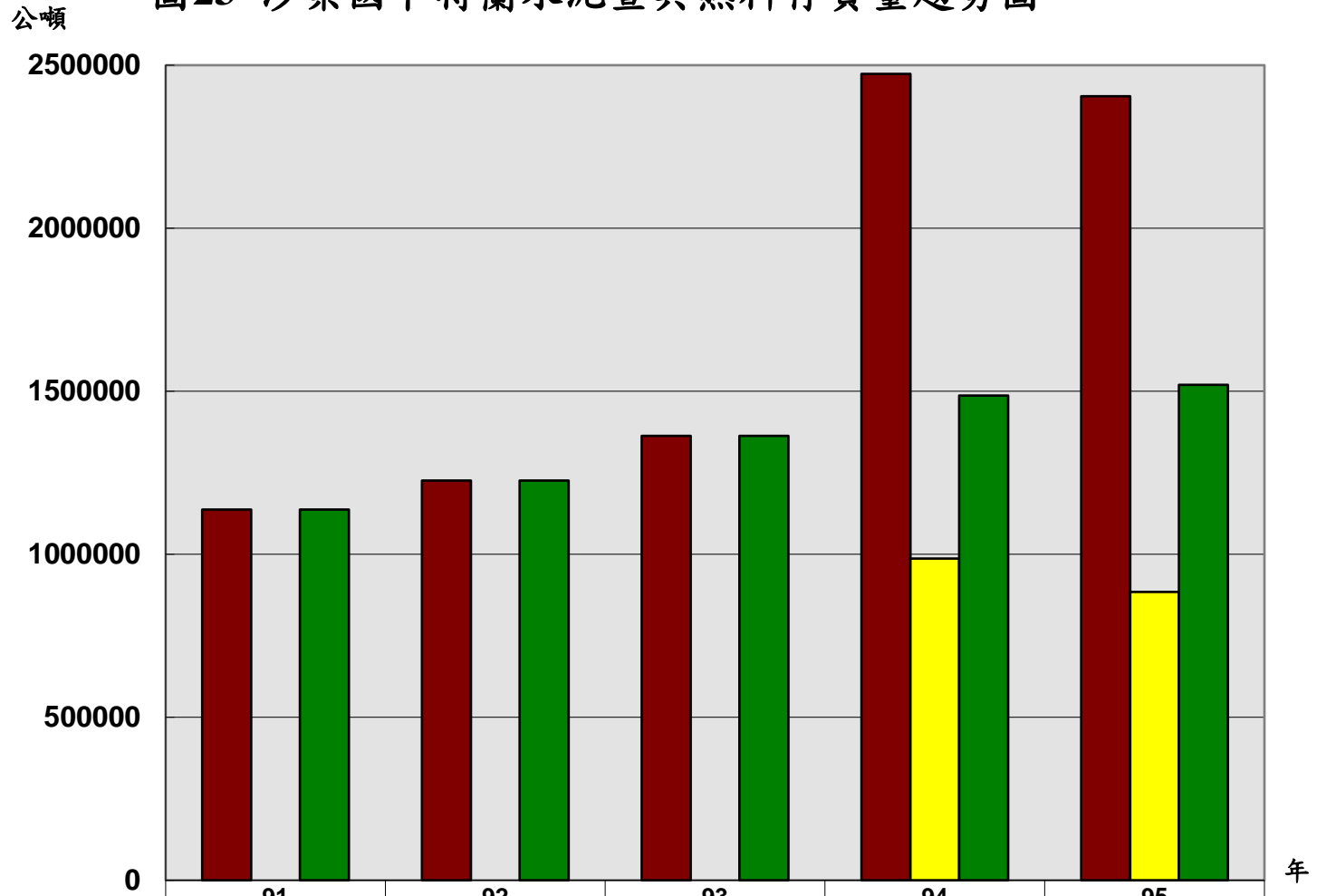
圖23 涉案國卜特蘭水泥暨其熟料存貨量趨勢圖
