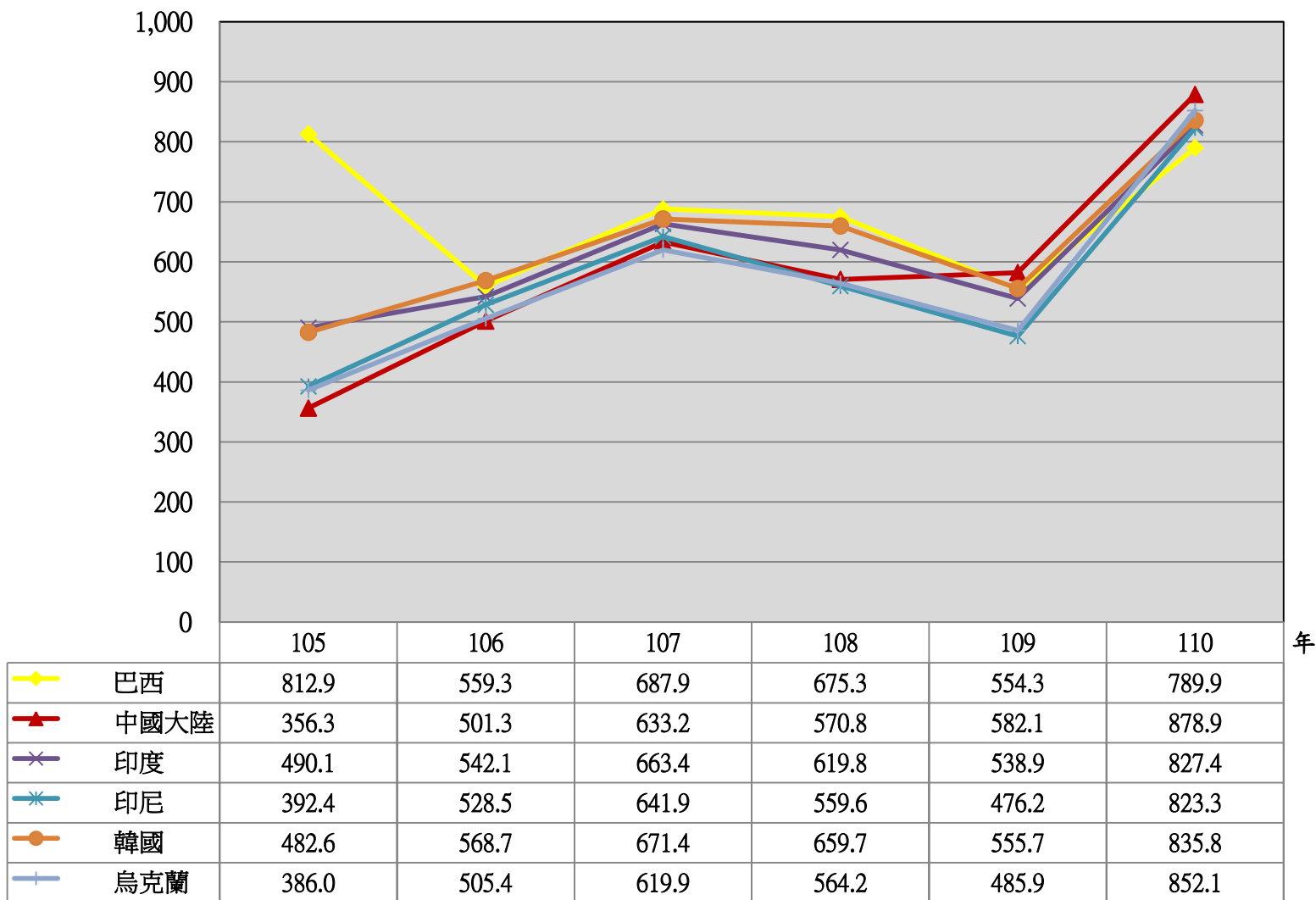
圖25 涉案國碳鋼鋼板產業平均外銷價格趨勢圖
