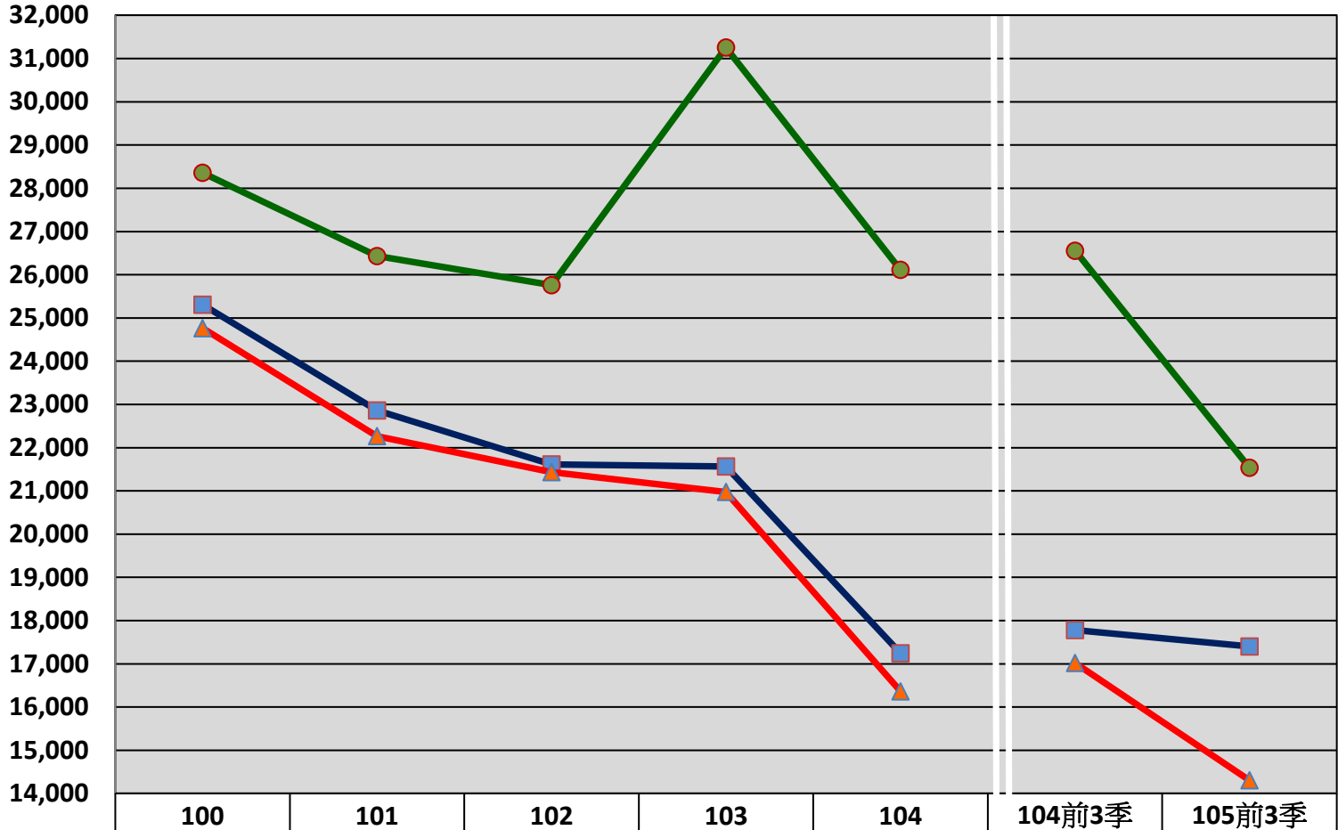
圖5 特定鍍鋅鋼品價格趨勢圖
