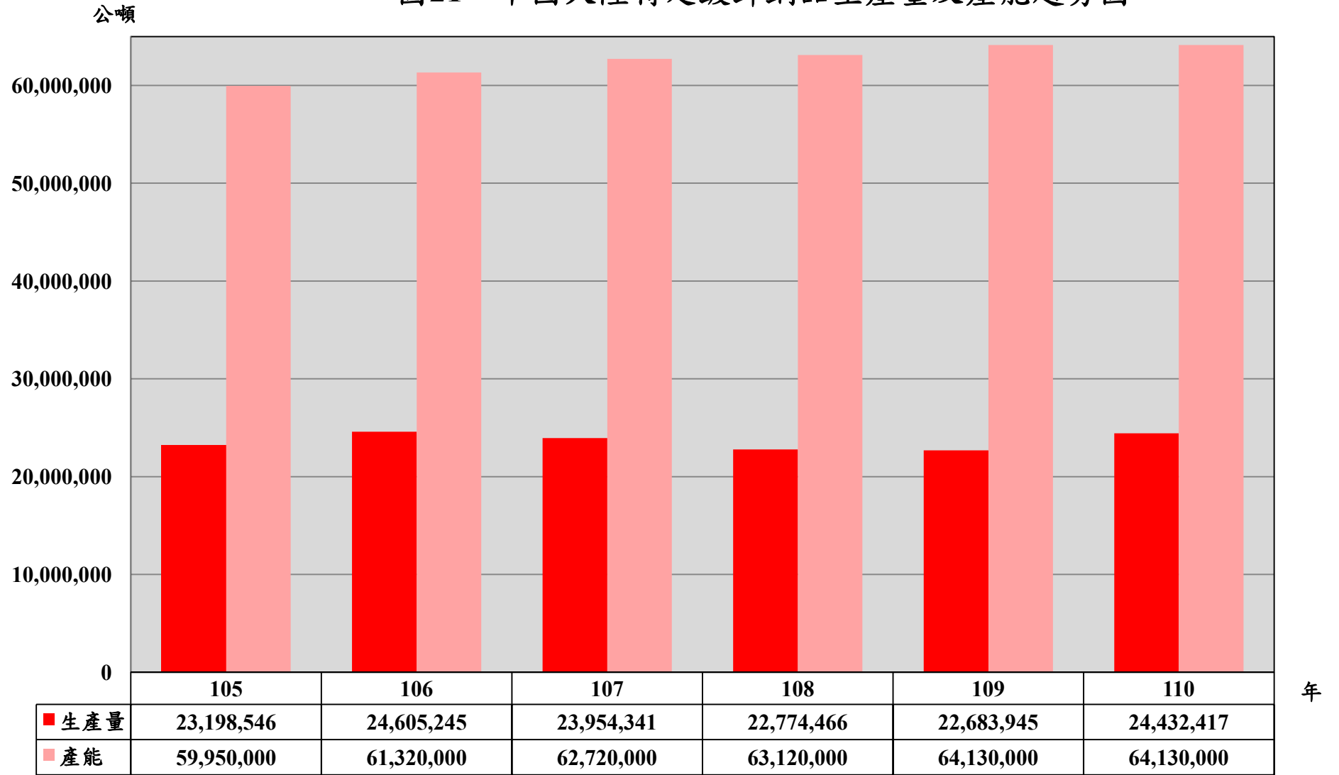
圖21 中國大陸特定鍍鋅鋼品生產量及產能趨勢圖
