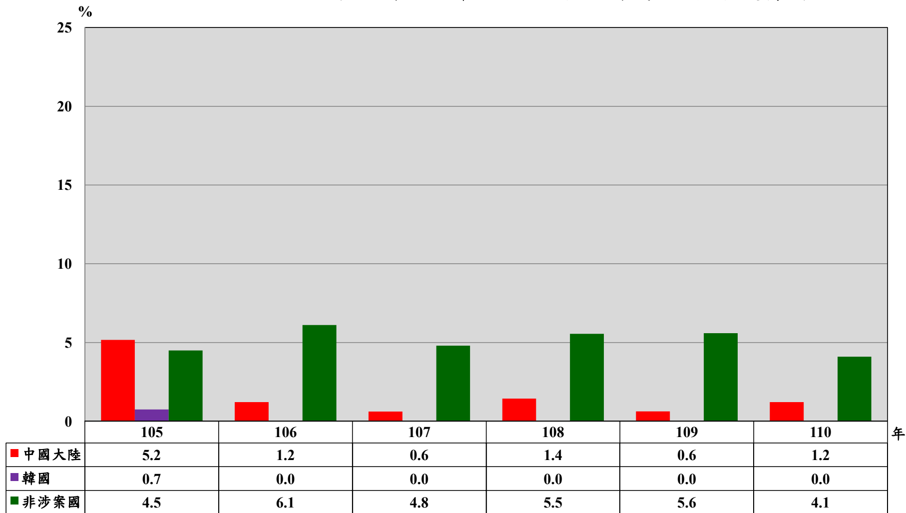
圖3 特定鍍鋅鋼品進口量相對我國生產量趨勢圖
