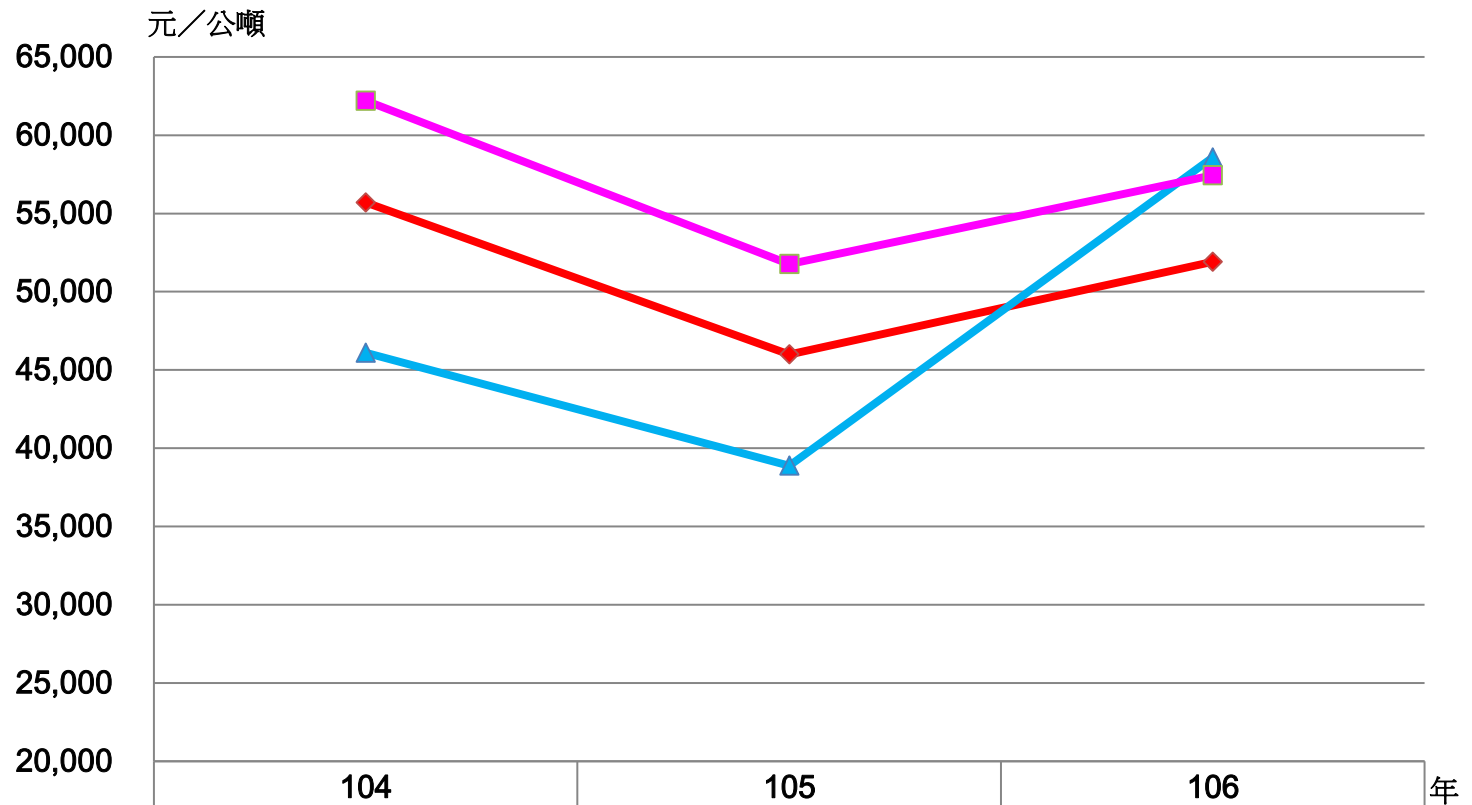
圖 5 特定不銹鋼熱軋鋼品價格趨勢圖
