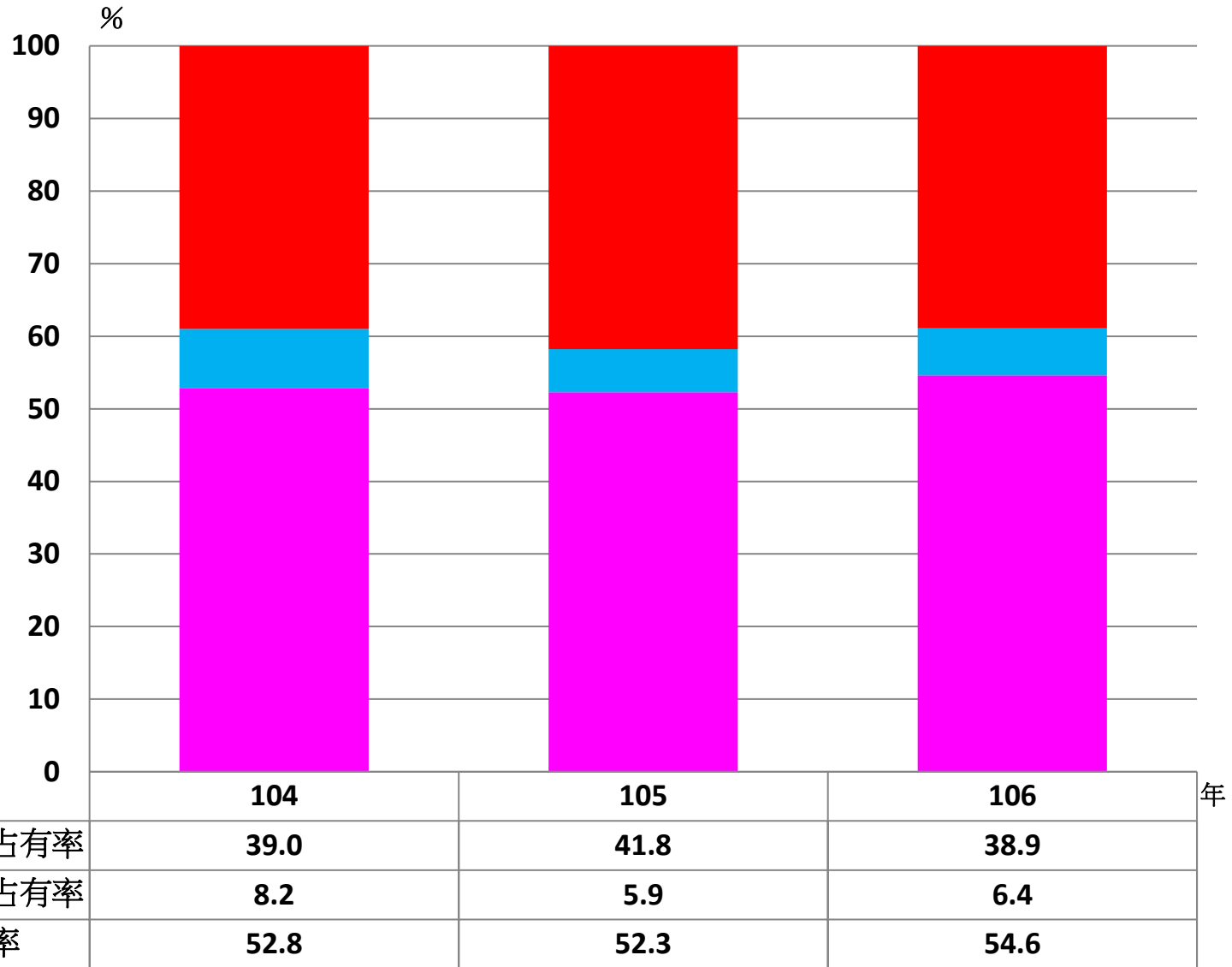
圖 4 特定不銹鋼熱軋鋼品進口量相對我國消費量趨勢圖
