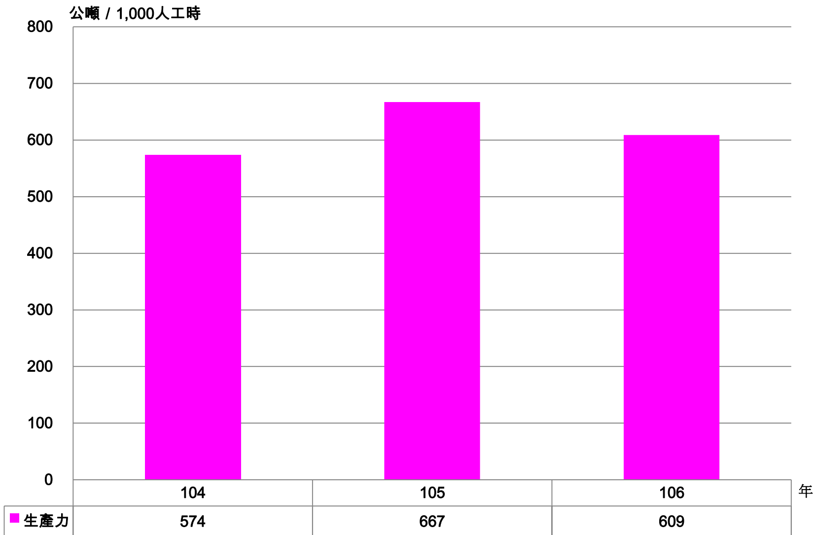
圖7 我國特定不銹鋼熱軋鋼品產業生產力趨勢圖
